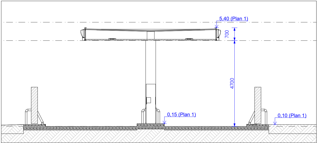
1:100 Snitt A
